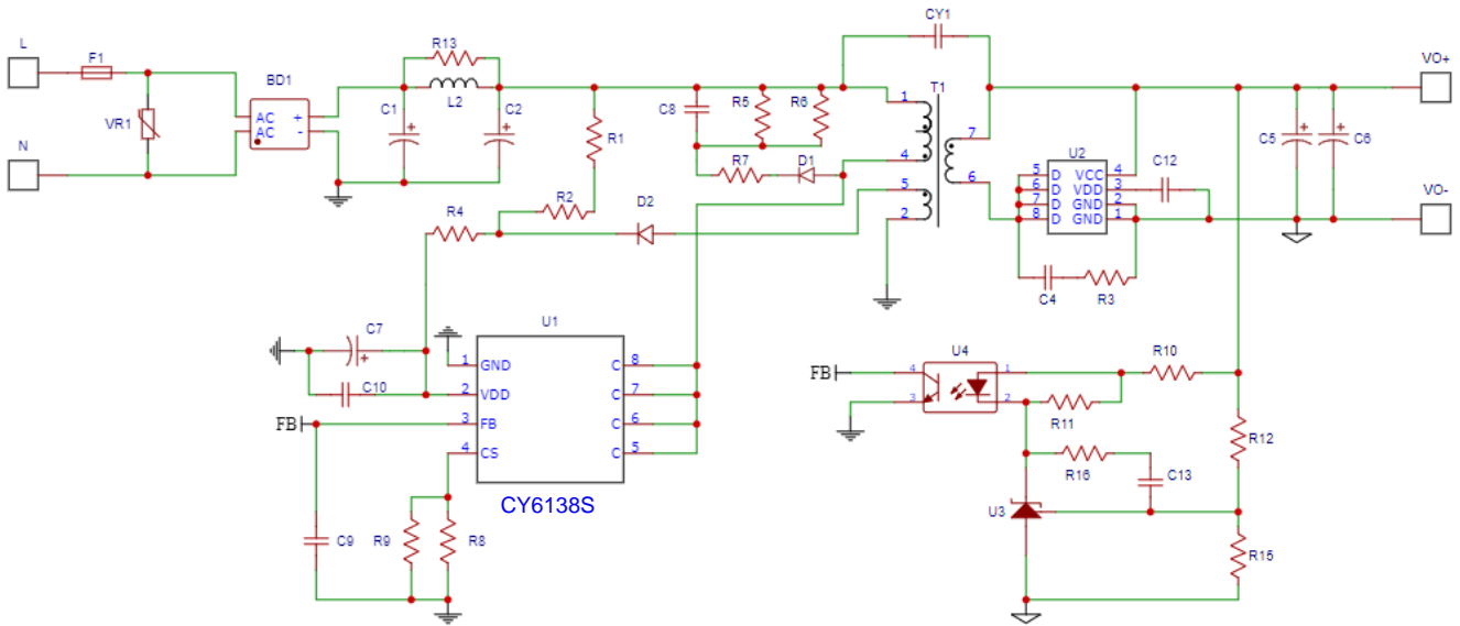
图2. CY6138S+同步整流芯片设计参考电路图 (90~265Vac输入，12V1.5A输出)
