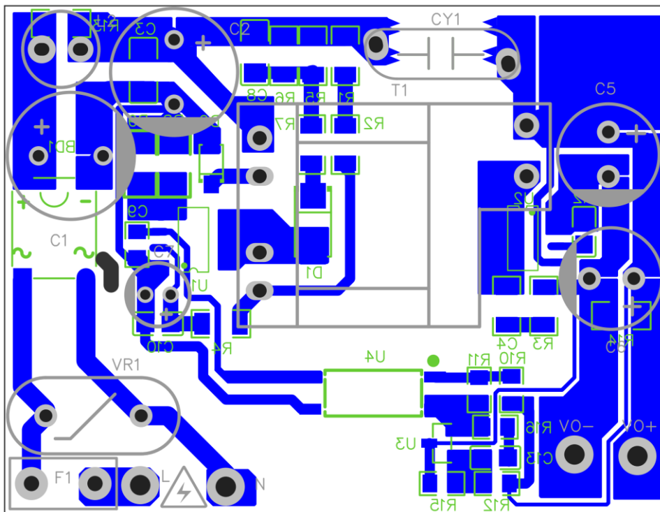
图3. CY6138S+同步整流芯片设计参考PCB Layout (90~265Vac输入，12V1.5A输出)
